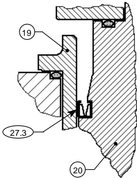
Tipo UC – Sello Dinámico en U
