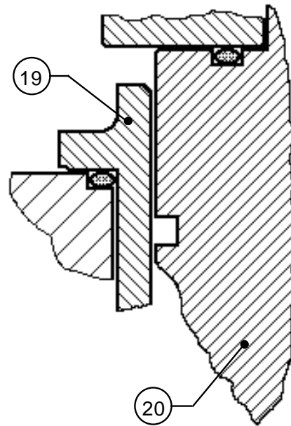
Tipo NO – No Sello Dinámico
