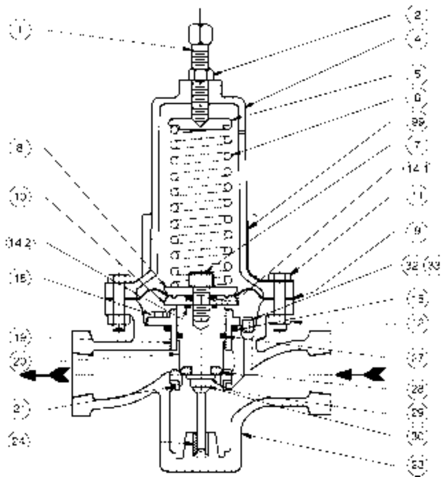
MODELO DA5 Diafragma Compuesto Dirección de Flujo Reverso FTO
