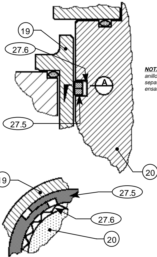
Tipo PR – PRA Sello Dinámico
