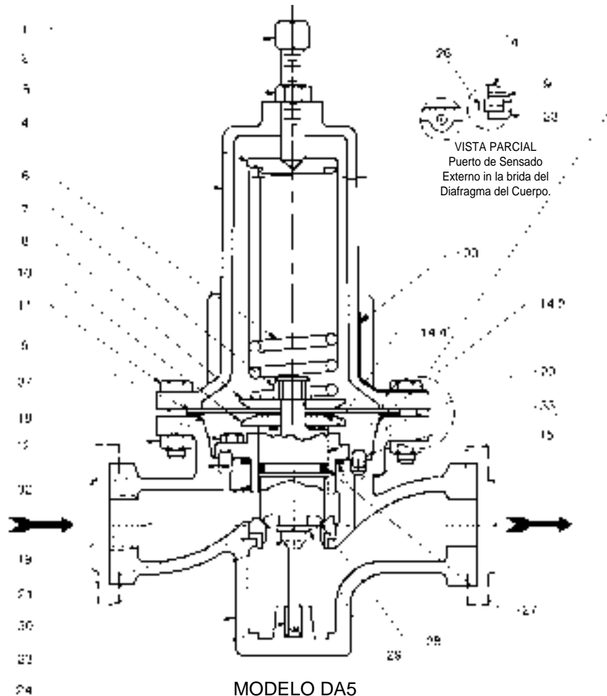
MODELO DA5 Diafragma Metálico Dirección de Flujo Estándar - FTC
